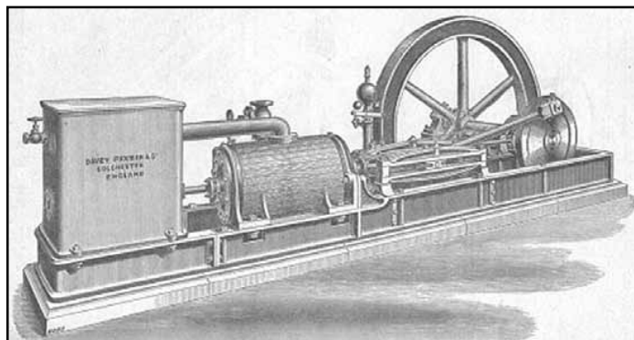
Máquina de bombeo de clase C, Davey, Paxman and Co., igual a la traída a Villanueva en 1891.
